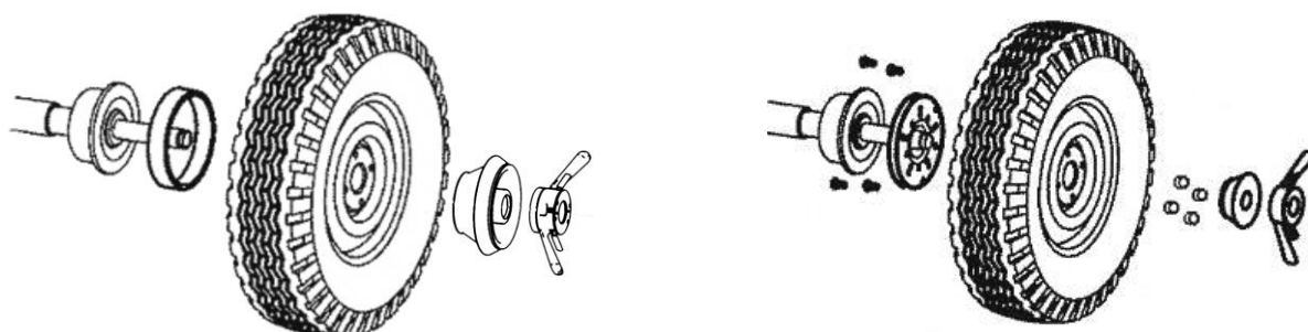
г – конус двусторонний Ø108...174 с кольцом
