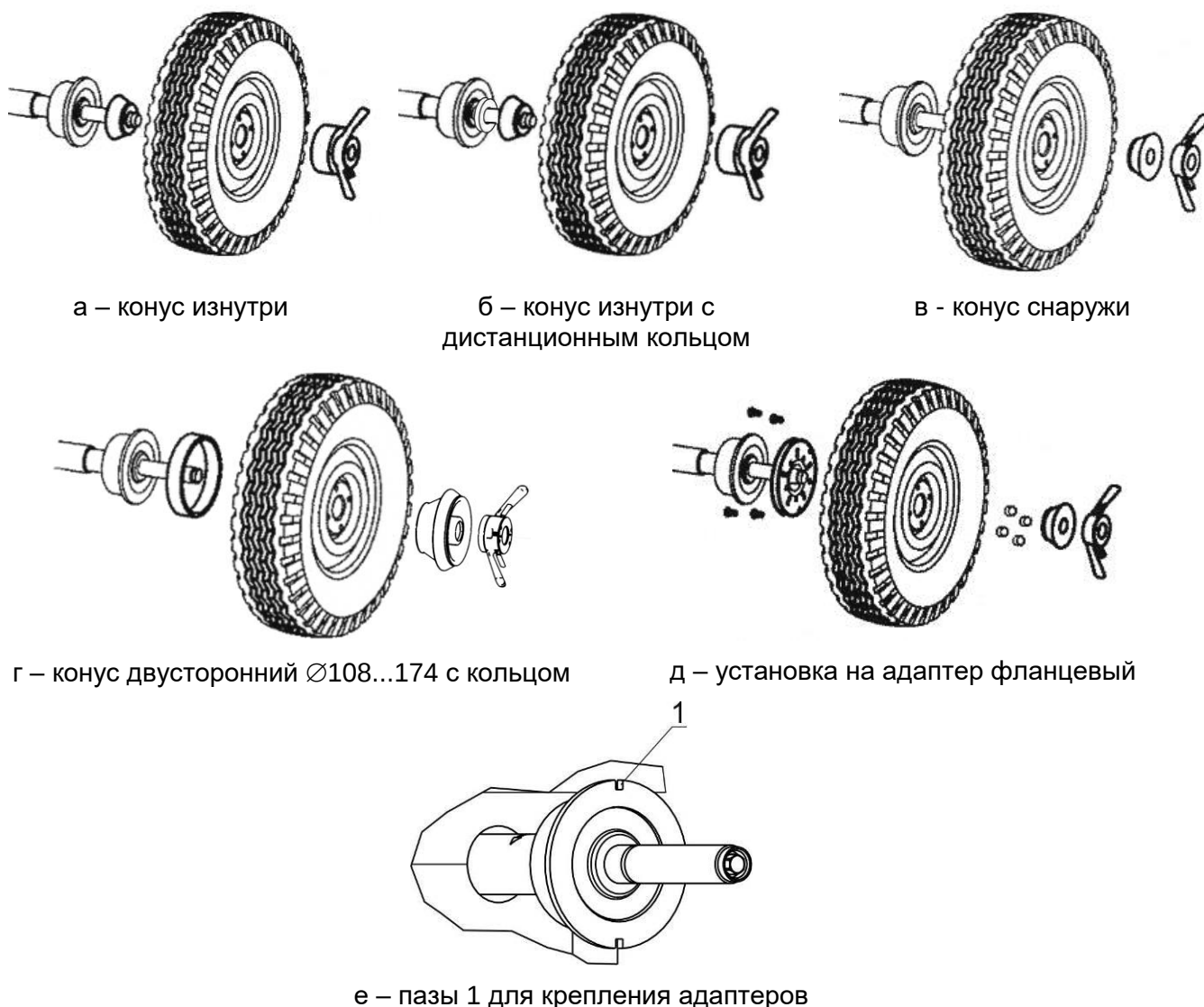
Рисунок 5.3 – Установка колеса
