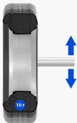
Влияние статического дисбаланса
