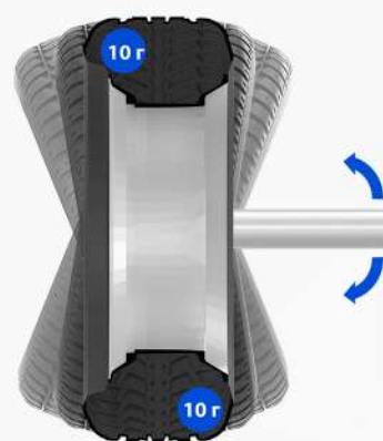
Влияние моментного дисбаланса
